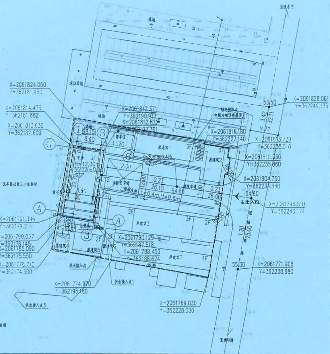
总平面图 1:500
